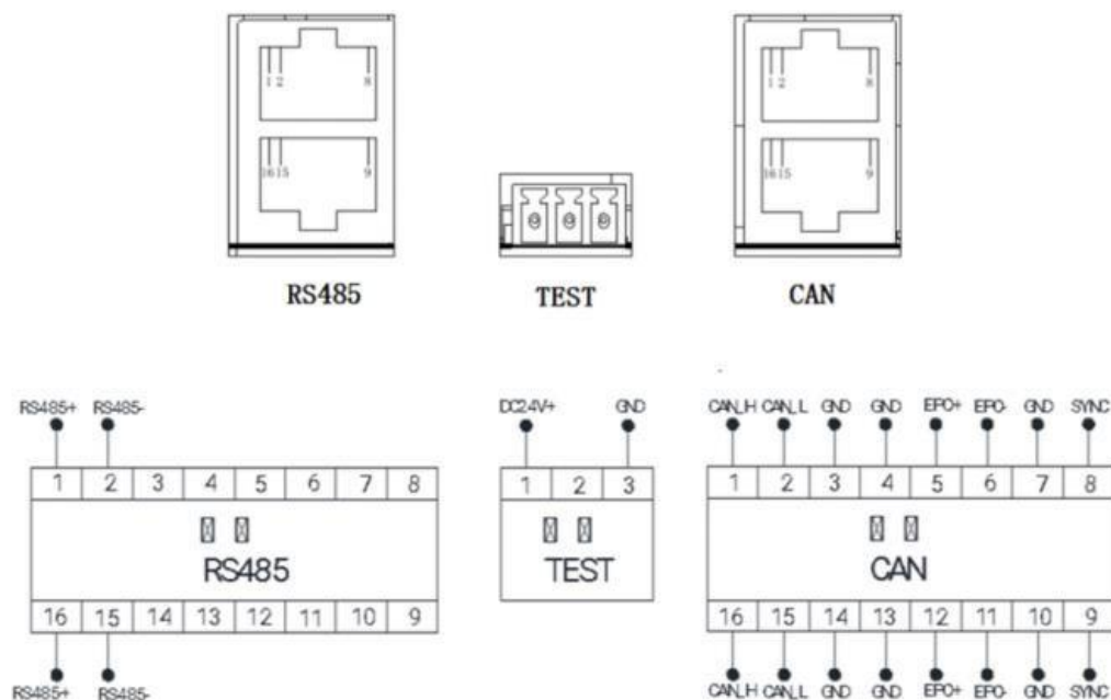
Rysunek 7. Wejścia sterownicze RJ45
