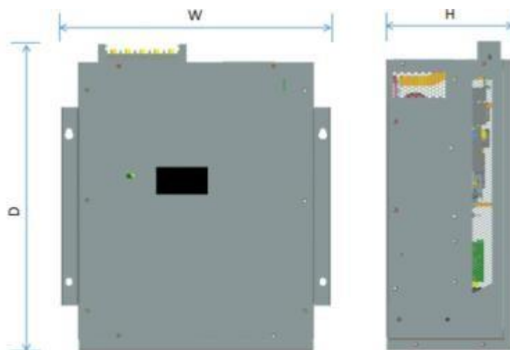
Rysunek 2. Widok kompensatora
